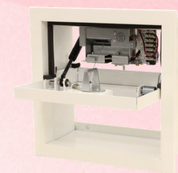
排煙口
