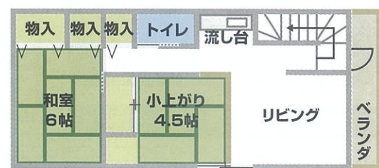
2階 平面図
